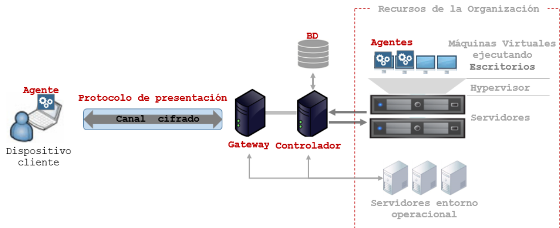
Figura 1: Arquitectura VDI con escritorios virtuales
