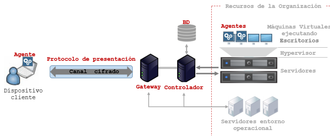
Figura 1: Arquitectura VDI con escritorios virtuales
