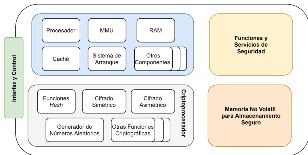
Figura 2. Arquitectura general de HSM.
