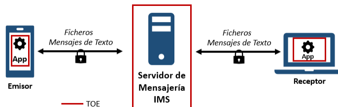
Figura 1: Caso de uso 1 - Arquitectura cliente-servidor
