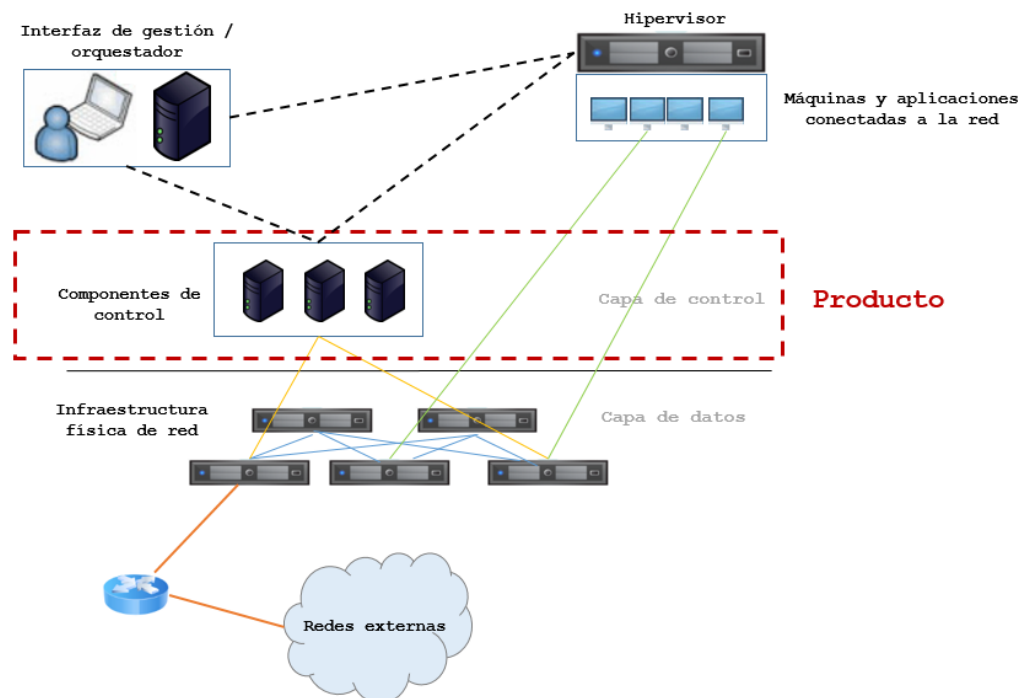
Figura 1: Caso de uso 1- Software controlador
