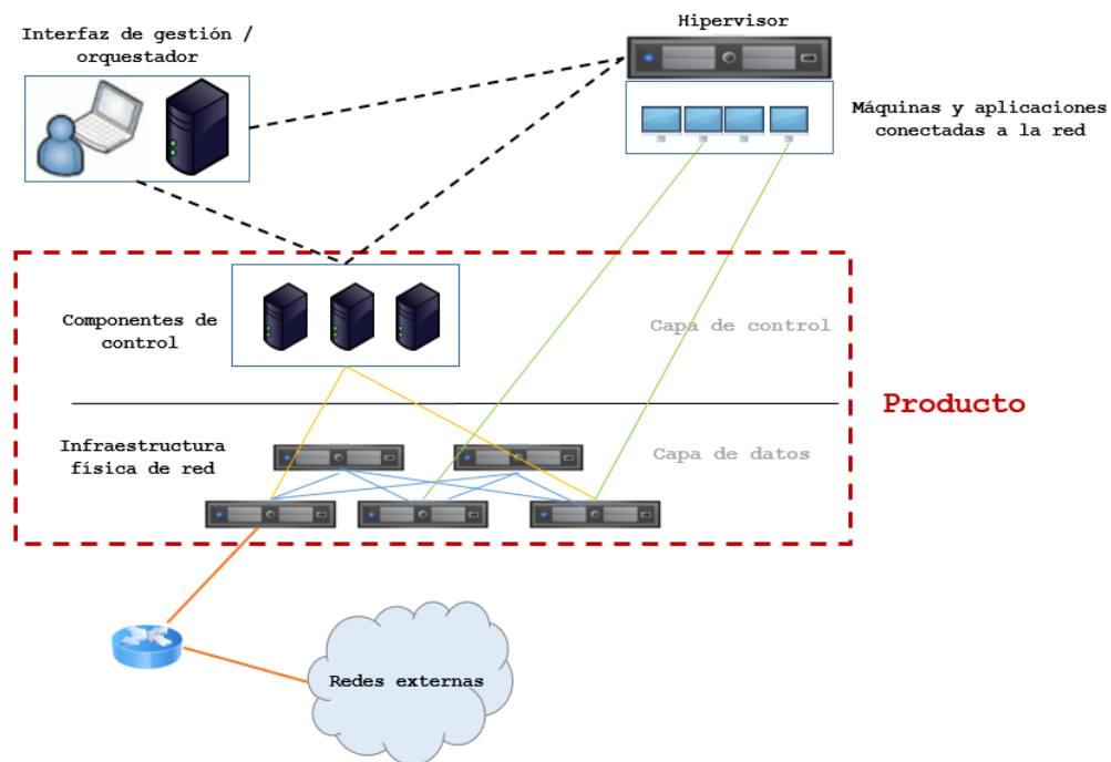
Figura 2: Software controlador e infraestructura hardware
