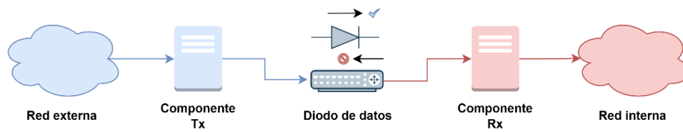
Figura 1: Caso de uso 1 - Flujo de entrada hacia la red interna
