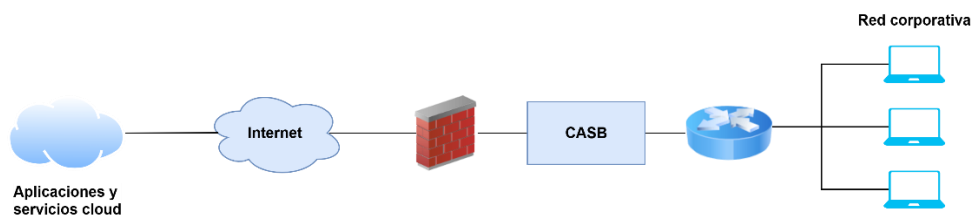
Figura 2: Caso de uso 2 - Modo proxy (online)
