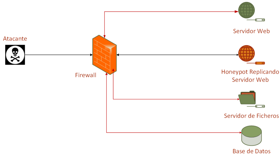
Figura 3: Caso de uso 3 - Replicación del servicio
