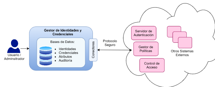
Figura 1: Caso de uso 1 - Gestor de identidades con almacenamiento propio
