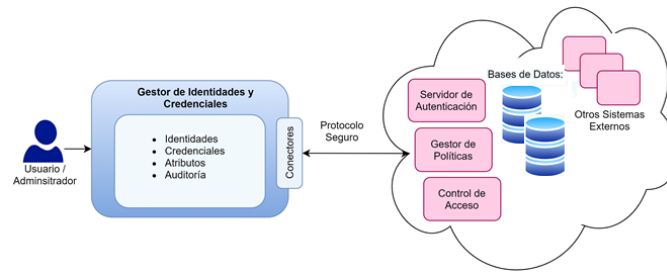
Figura 2: Caso de uso 2 - Gestor de identidades sin almacenamiento propio
