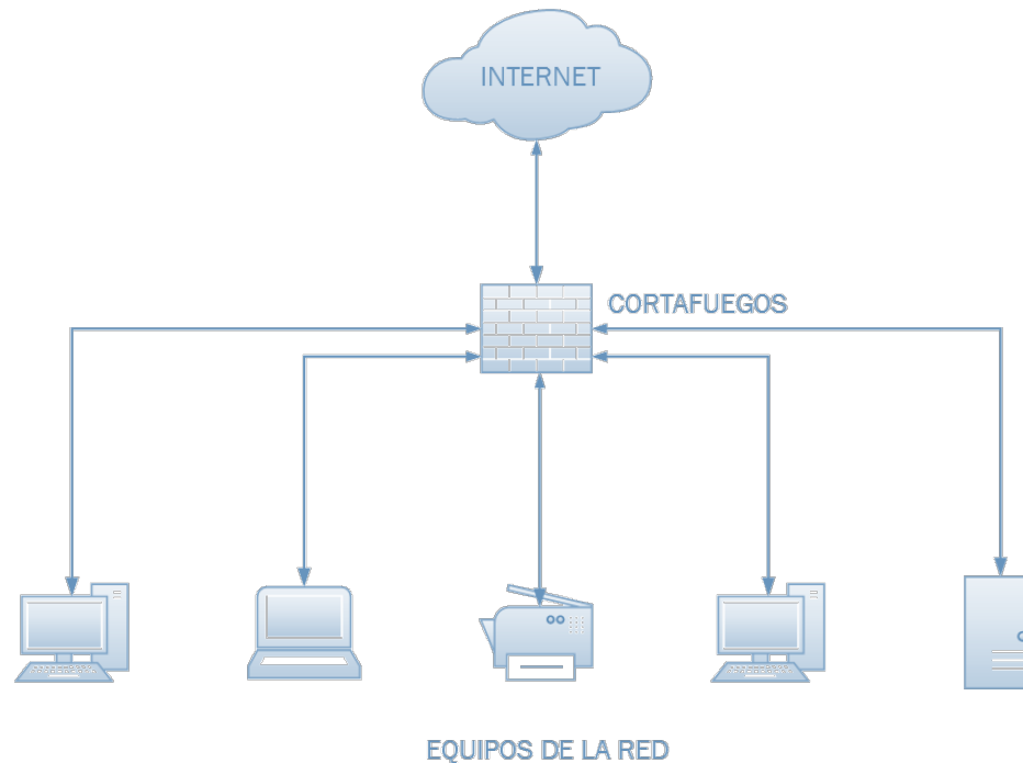
Figura 1 - Ejemplo de Caso de uso 1-Dispositivo frontera
