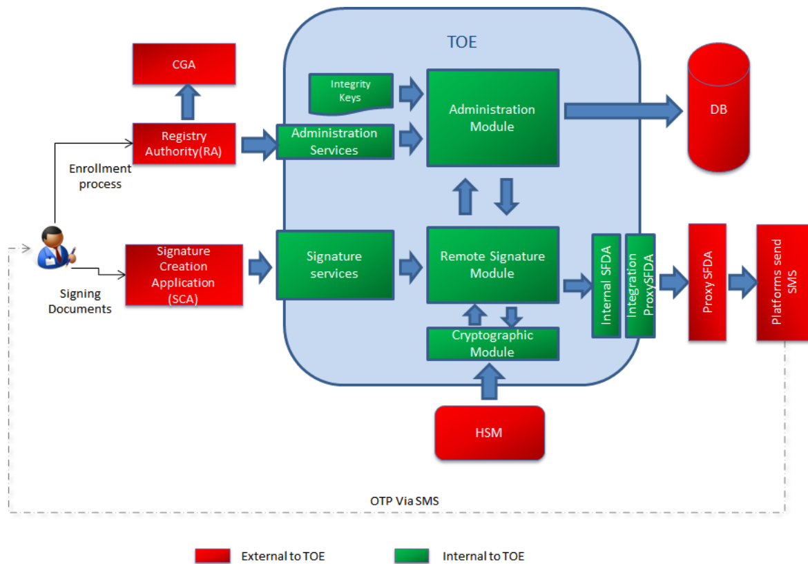
Ilustración 1: Arquitectura lógica del SIAVAL SafeCert Manager
