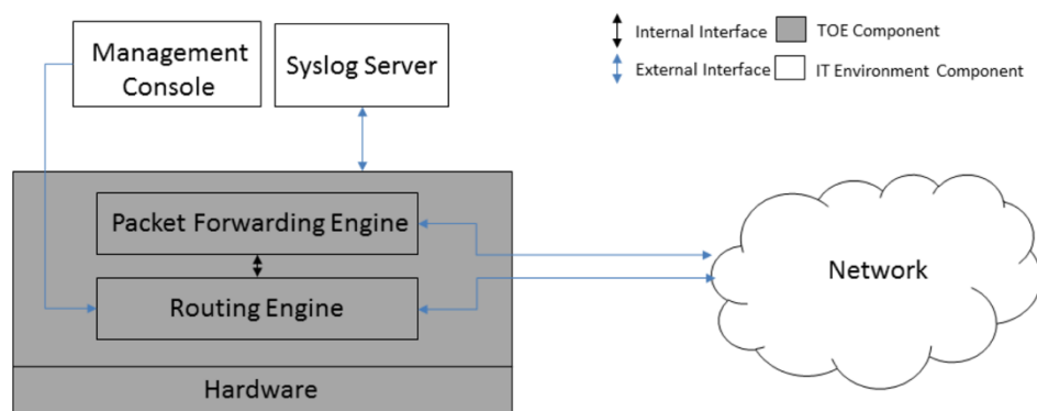
Figura 1 Arquitectura Física de dispositivos EX4100, EX4100-F, EX4400
