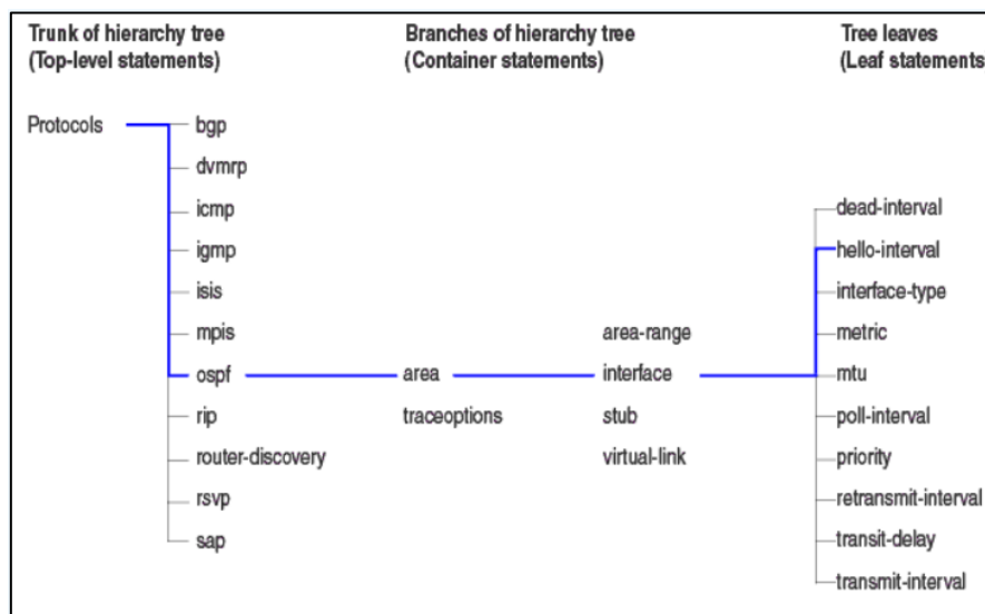
Figura 1 - Ejemplo de jerarquía de sentencias de configuración
