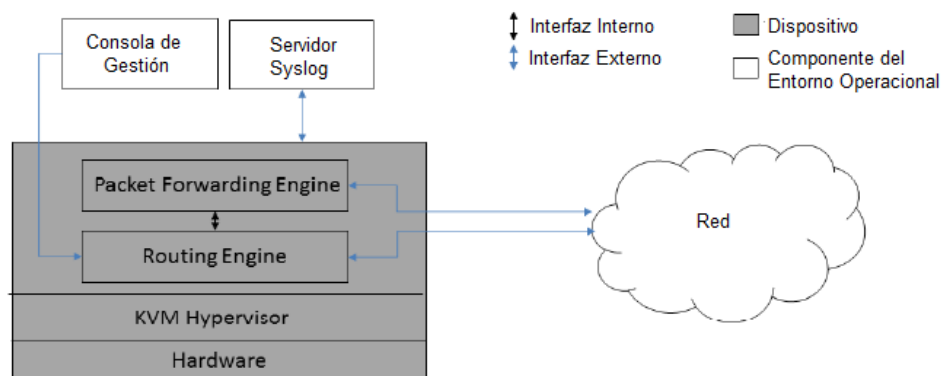
Figura 1- Arquitectura Física del dispositivo ACX5448
