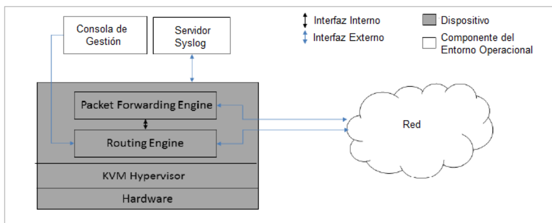
Figura 1 - Arquitectura física de dispositivos SRX1500, SRX1600, SRX2300, SRX4100, SRX4200, SRX4300, SRX4600, SRX5400, SRX5600, SRX5800
