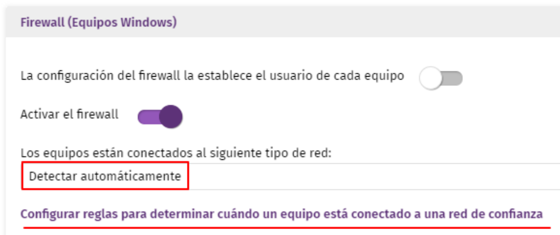
Figura 28: Firewall (Equipos Windows) > Configurar reglas para determinar cuándo un equipo está conectado a una red de confianza
