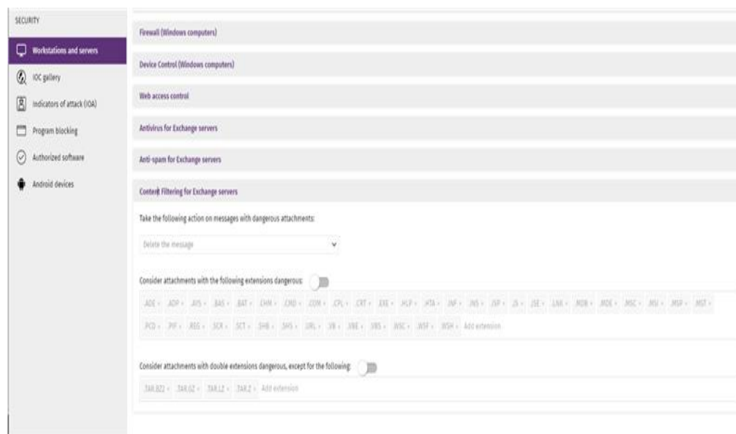
Figura 35: Menú Configuración > Estaciones y Servidores > Filtrado de contenidos para servidores Exchange
