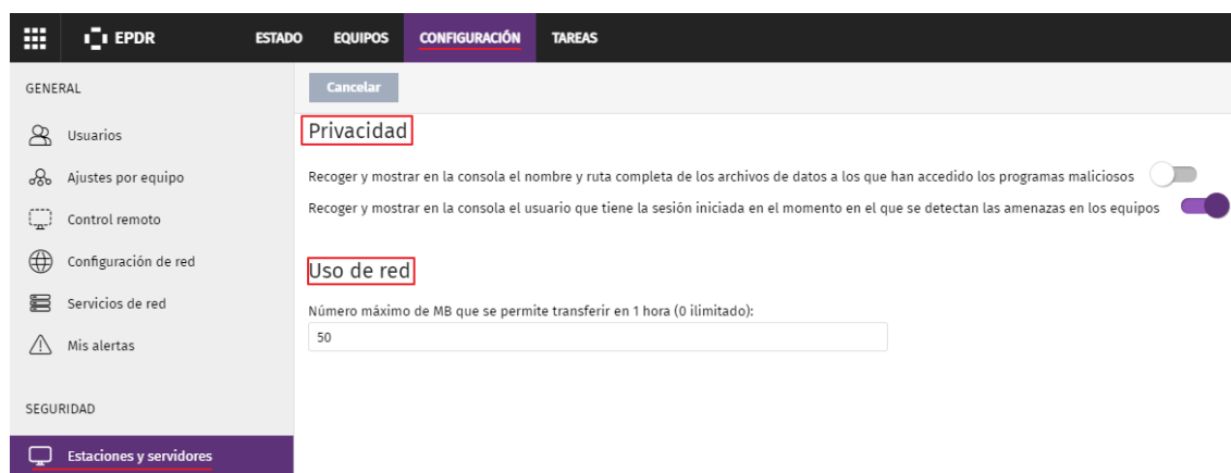
Figura 50: Menú Configuración > Estaciones y servidores
