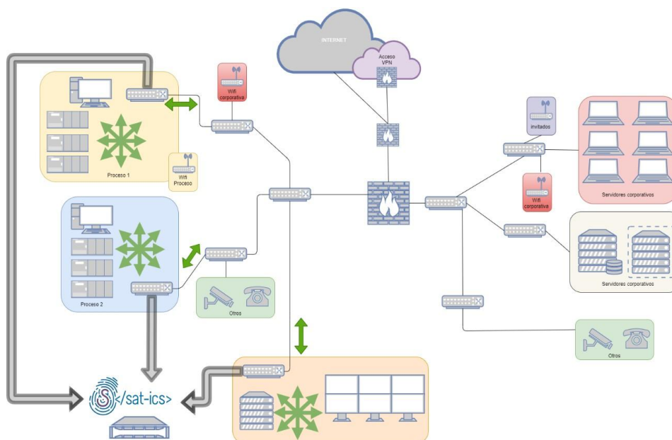
Figura 3. Esquema de monitorización interna
