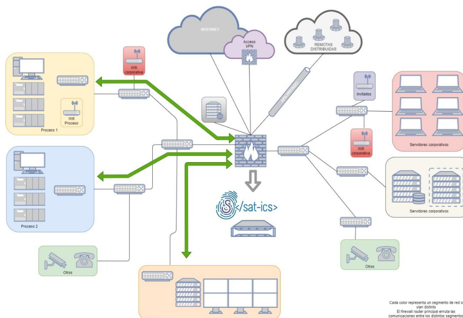
Figura 4. Esquema de monitorización perimetral
