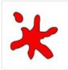
ollydbg
